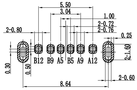
PCB板参考图
